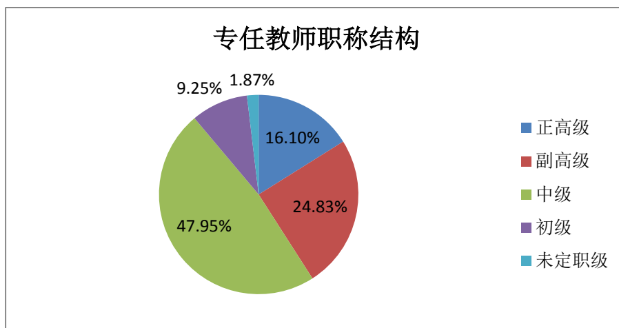
图 1 职称结构
